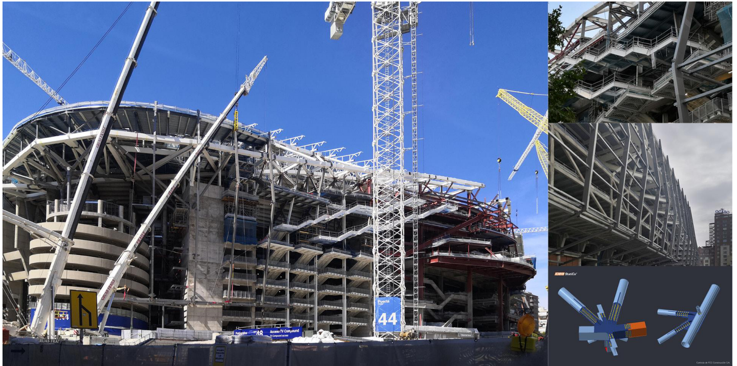
Edificio Este. Fachada y Estructura del videomarcador
